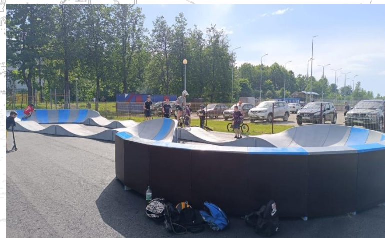
Установка памп-трека
